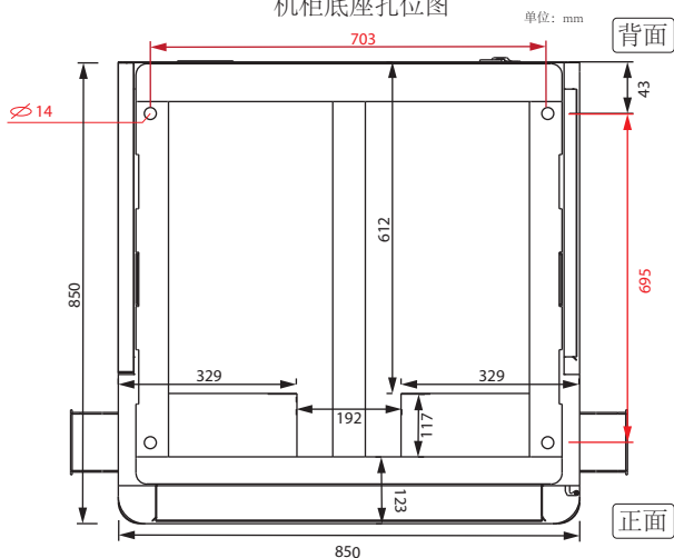
机柜底座孔位图
