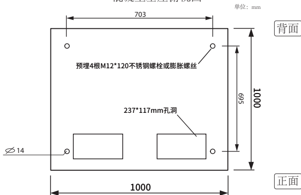
混凝土基座俯视图
