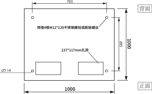
混凝土基座俯视图
