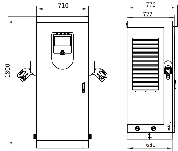
机柜正视图
