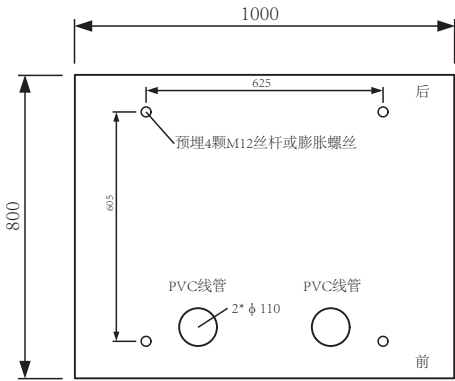
混凝土基座俯视图
