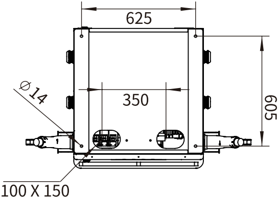
机柜底座孔位图
