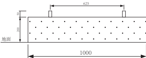
混凝土基座正视图
