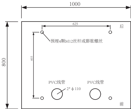
混凝土基座俯视图
