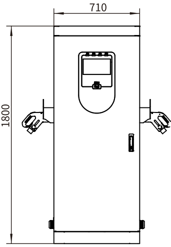
机柜正视图
