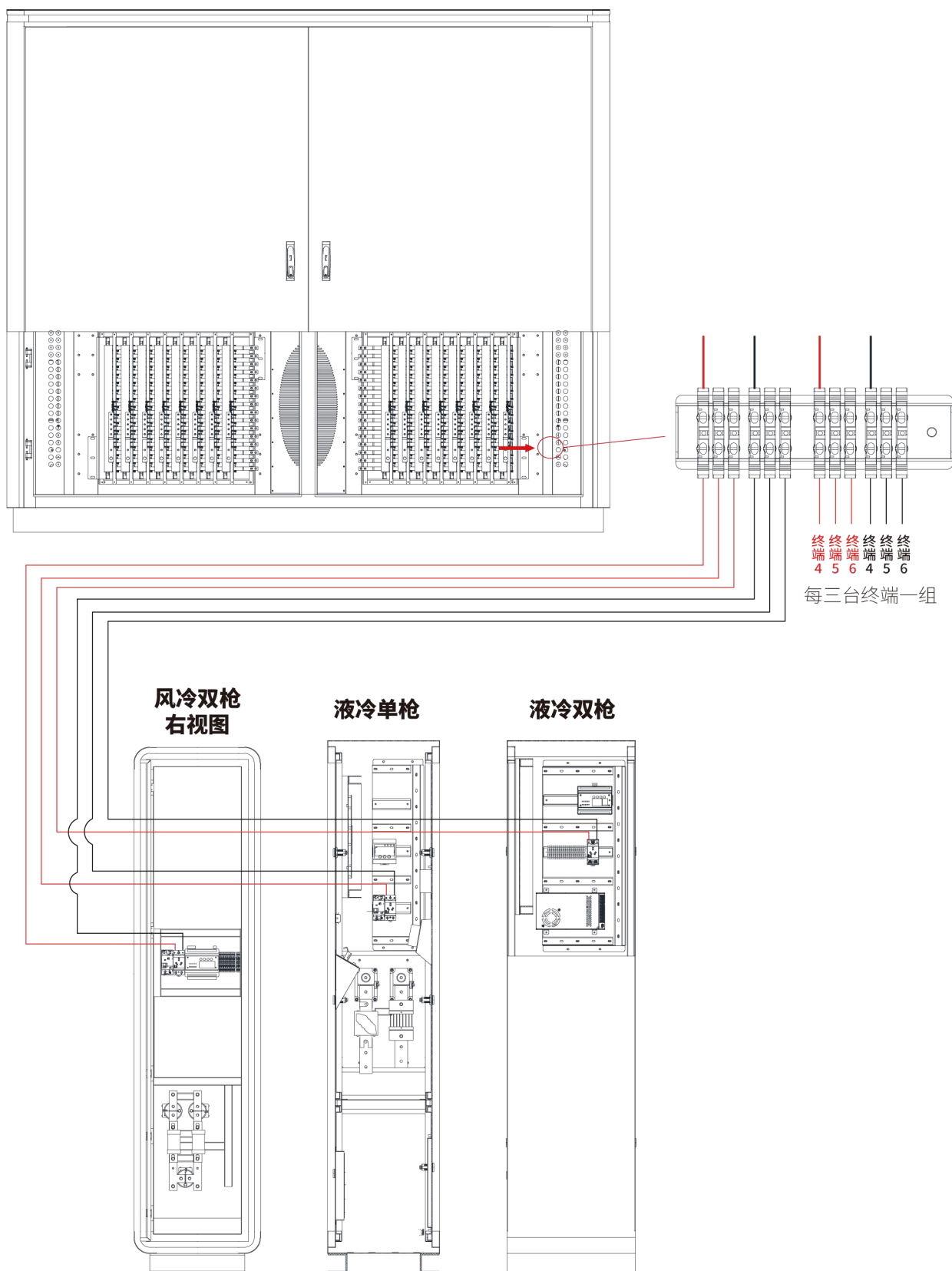
4、主机柜到终端 can 通讯线接线示意图
