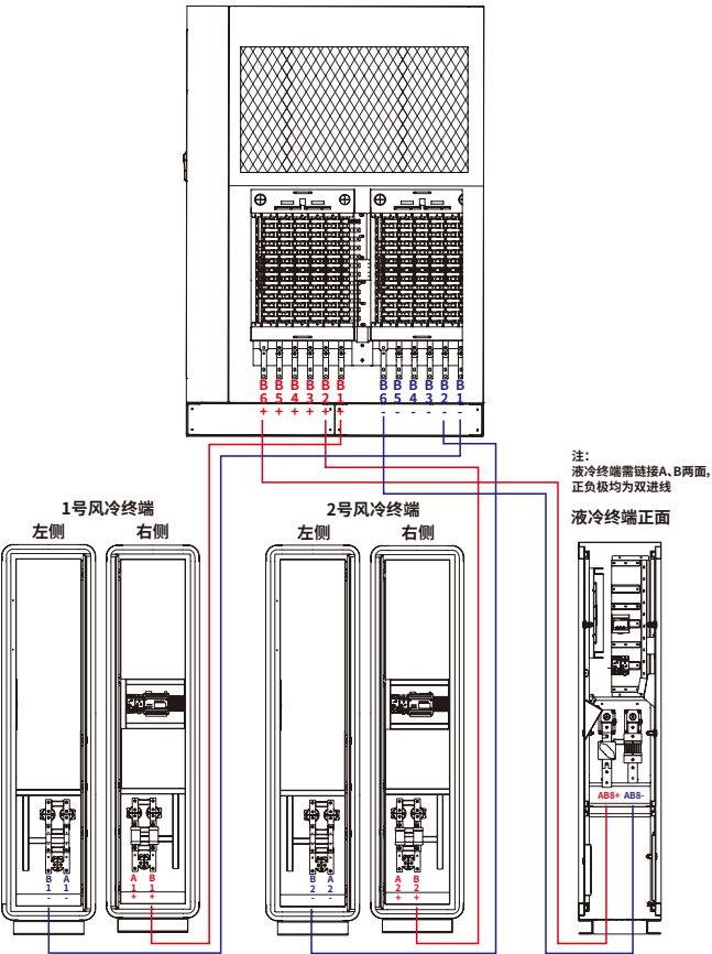
(B面终端接线详图)
