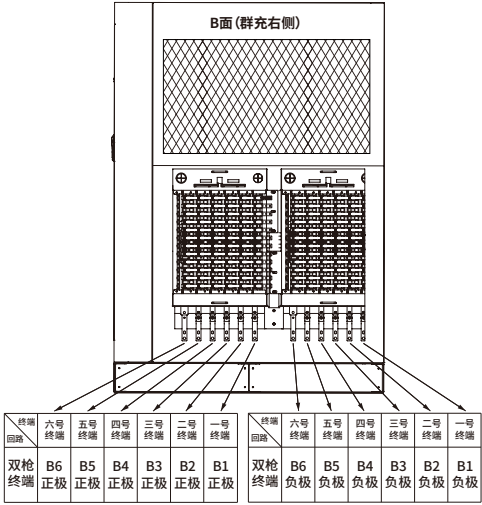
(B面终端接线总图)
