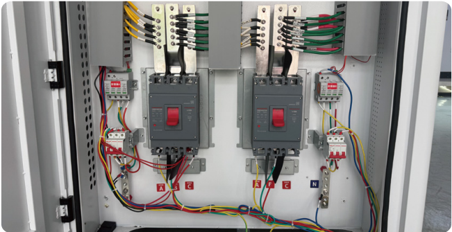
(正面机器内部实拍图)
