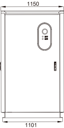
(群充主机机柜正视图)
