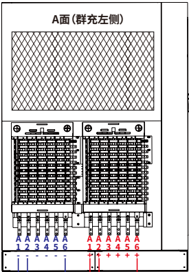
(A面终端接线详图)
