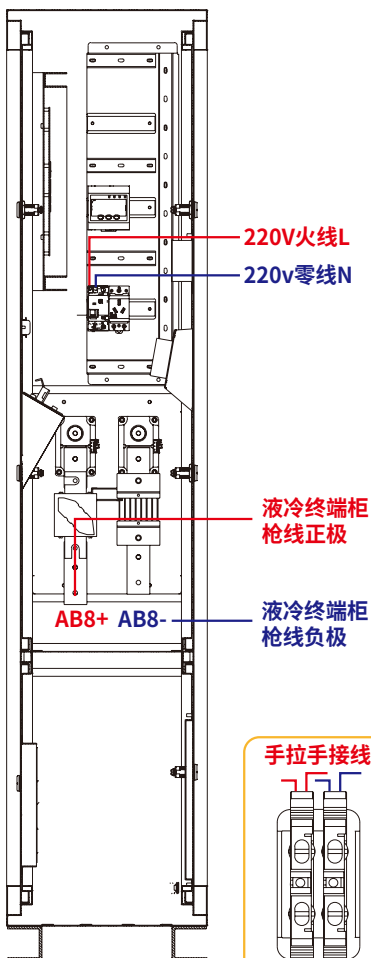
(液冷终端正面图)
