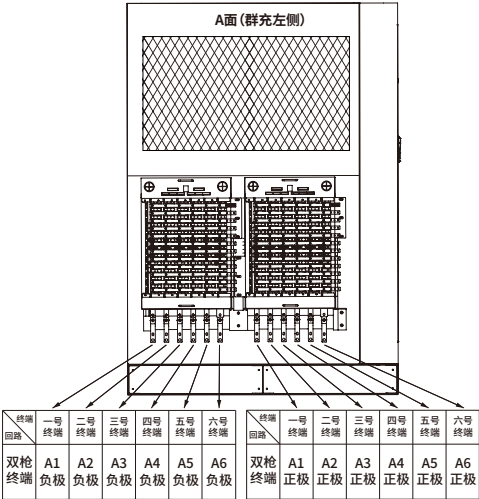
(A面终端接线总图)
