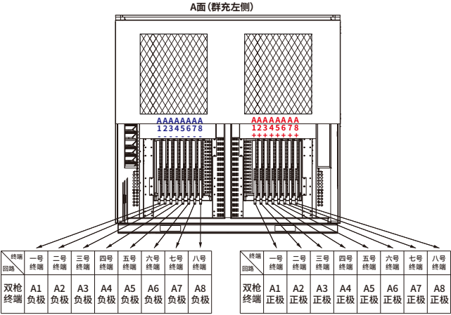
(A面终端接线总图)
