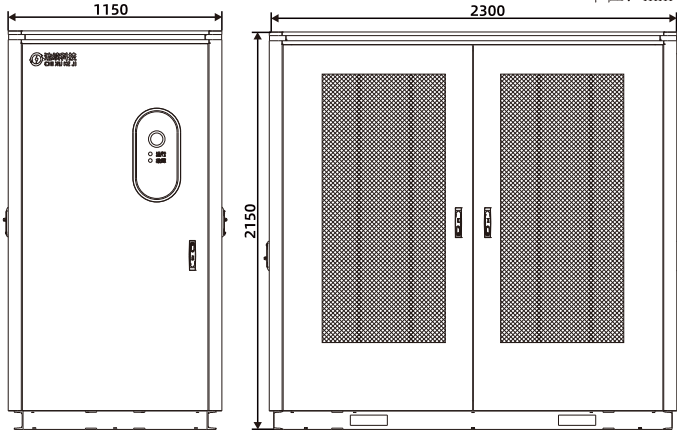
(群充主机机柜正视图)
