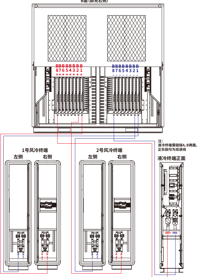
(B面终端接线详图) B面(群充右侧)
