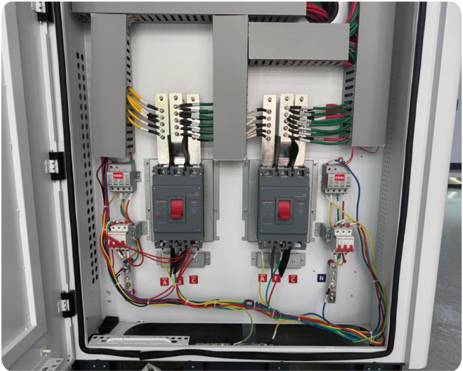
(背面机器内部实拍图)
