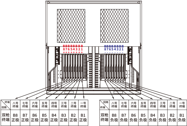
(B面终端接线总图) B面(群充右侧)
