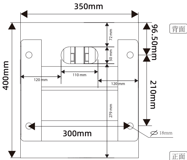
(风冷群充终端柜柜孔位图)
