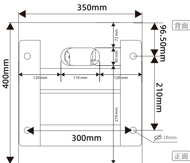
(液冷群充终端柜柜孔位图)
