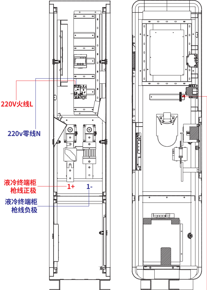
(液冷终端正面图)
