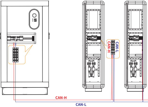
(风冷终端右侧)
