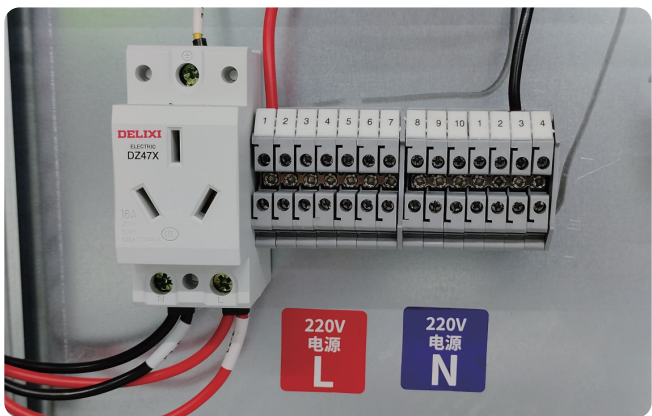
群充220V接电图
