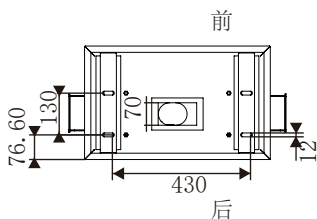
群充终端柜(风冷)柜孔位图
