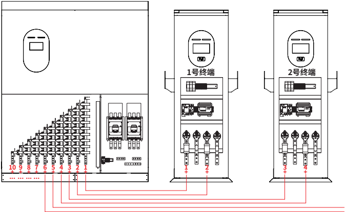
群充正极 (群充柜前面铜排) 接终端柜正极
