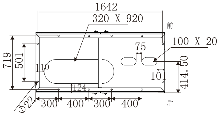
群充主机柜孔位图
