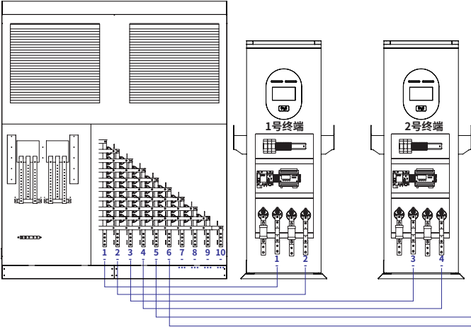
群充负极(群充柜背面铜排)接终端柜负极
