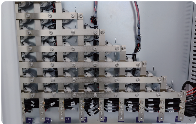
群充直流输出（枪线）负极图
