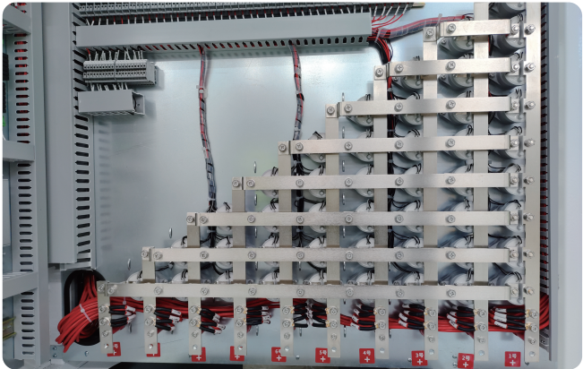
群充直流输出（枪线）正极图
