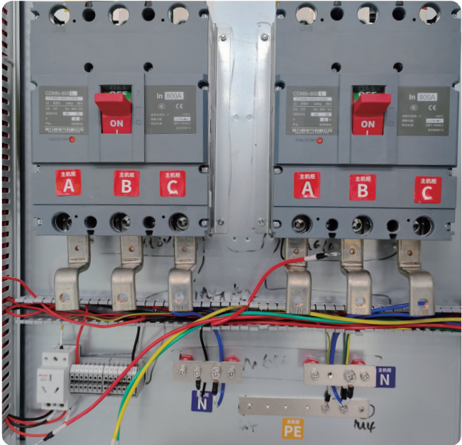
群充380V进线图
