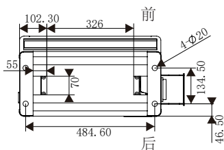
群充终端柜(液冷)柜孔位图
