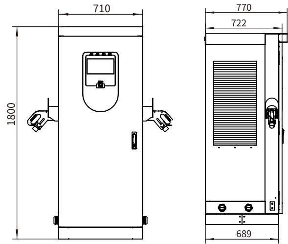
机柜正视图
