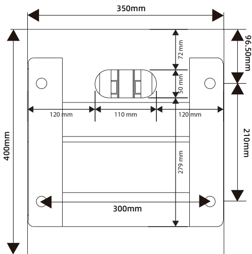
(风冷群充终端柜柜孔位图)
