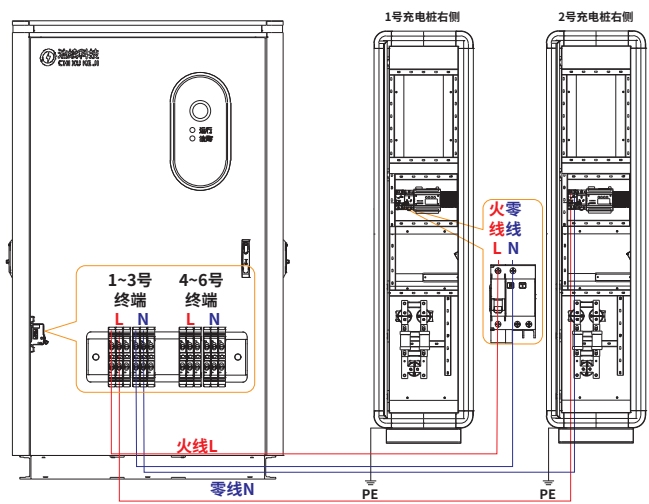
(线形接线示意图)
