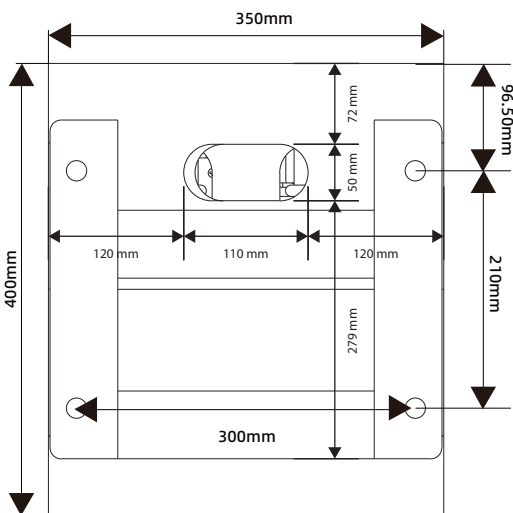
(液冷群充终端柜柜孔位图)
