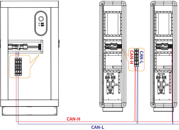
(风冷终端右侧)
