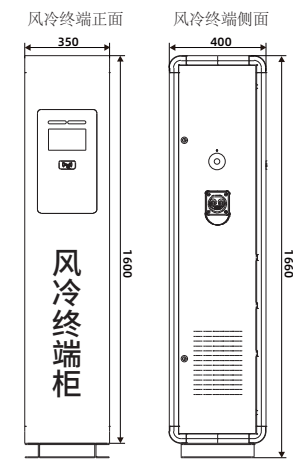
(风冷群充终端柜机柜尺寸图)
