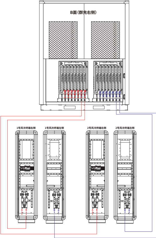
(B面终端接线详图)
