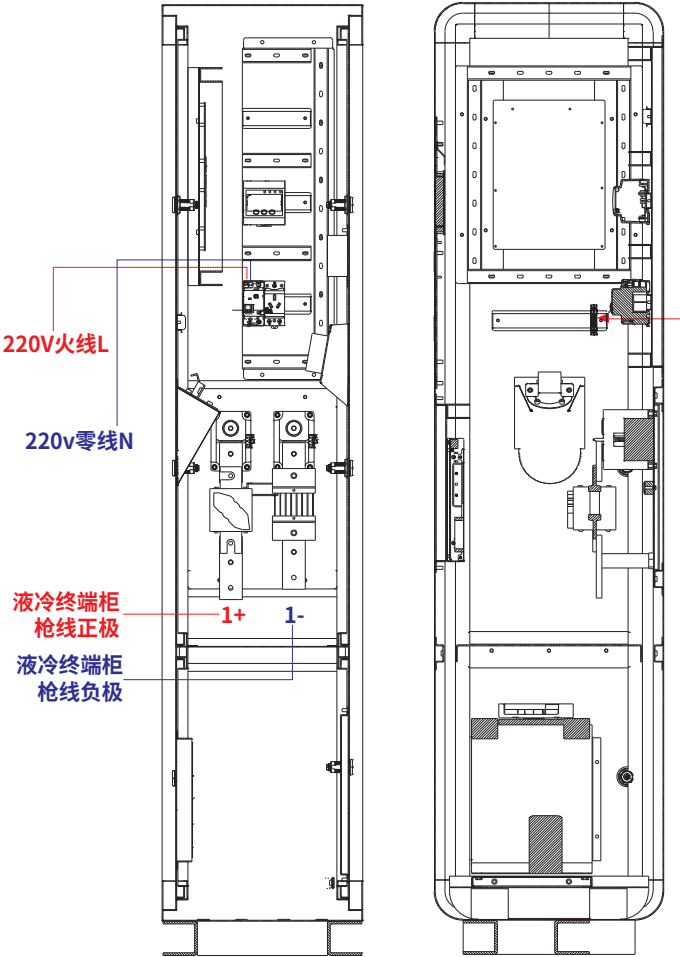
(液冷终端正面图)
