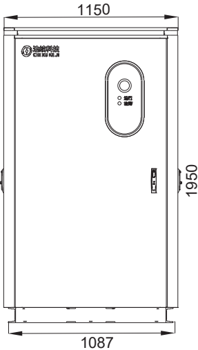
(群充主机机柜正视图)
