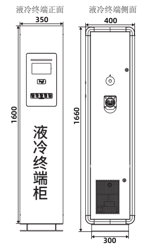
(液冷群充终端柜机柜尺寸图)
