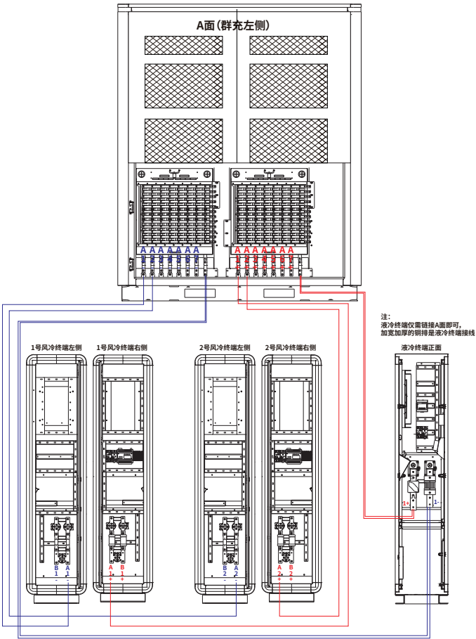
(A面终端接线详图)
