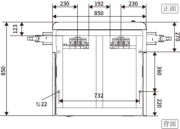
混凝土基座俯视图
