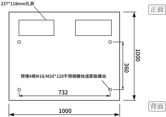
混凝土基座俯视图
