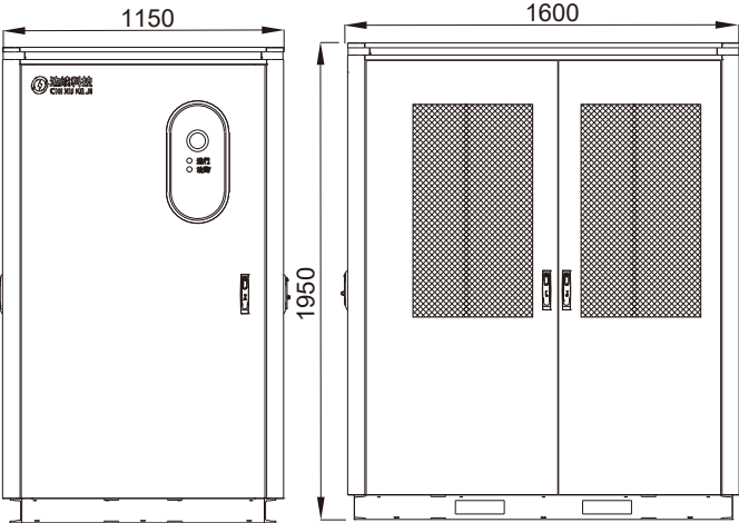
(群充主机机柜正视图)
